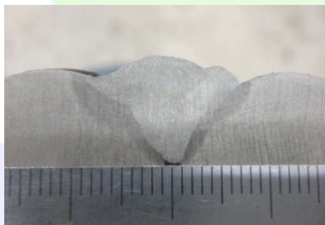
鋼の断面マクロ試験
