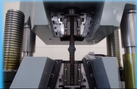
ガス圧接の引張強度試験
