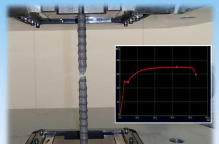
素材鉄筋の引張強度試験
