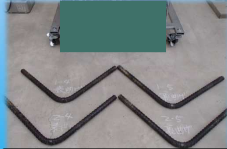
金属材料曲げ試験
